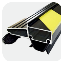
PERFIL INFERIOR SUPER REDUZIDO escalón reducido profil inférieur super reduced low threshold
