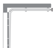
PADIEIRA REDUZIDA dintel reducido lindeau avec ressort arrière reduced lintel
